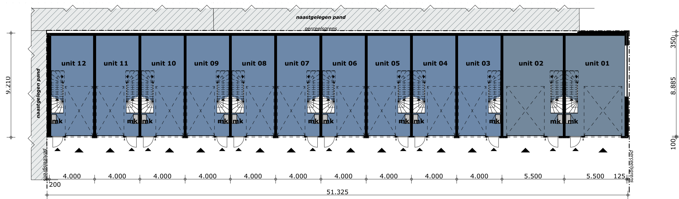
BEGANE GROND
