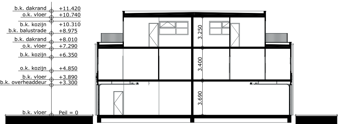
DOORSNEDE B-B
