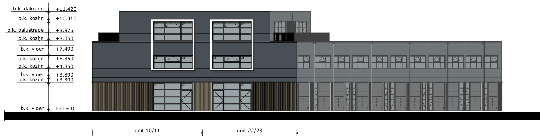
NOORD-OOST GEVEL
